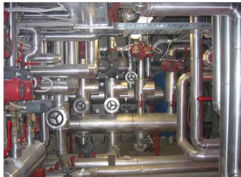
Sottocentrale termofrigorifera zona "cementi" - Special Plant
