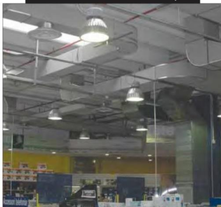
Distribuzioni aeree - Aeraulic System
